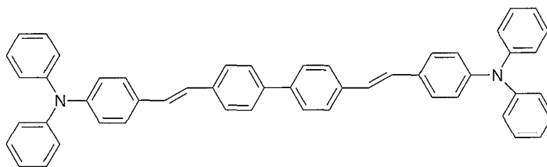
DSA amine
