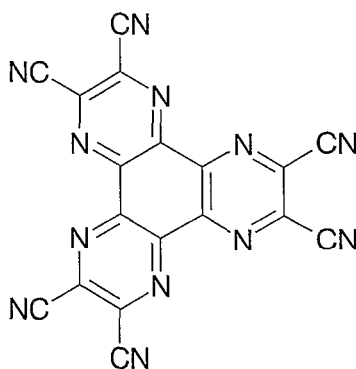
Hexanitride hexaazatriphenylene
