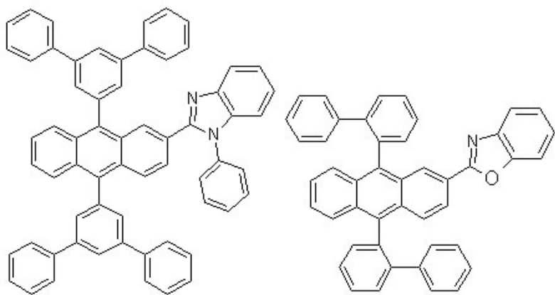
[화학식 3-7] [화학식 3-8]
