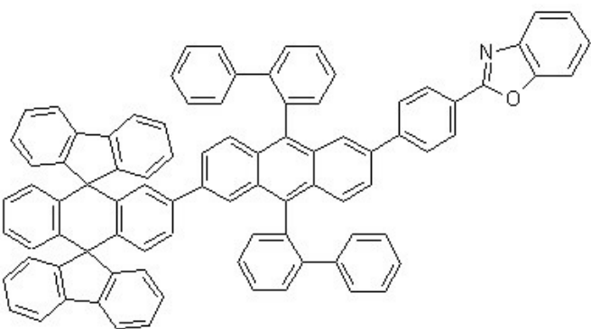
[화학식 1-16]
