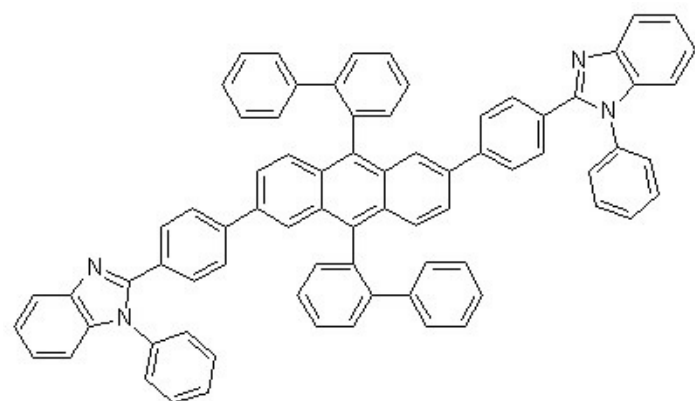
[화학식 2-3]
