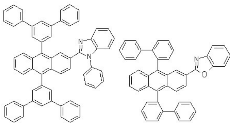
[화학식 3-7] [화학식 3-8]
