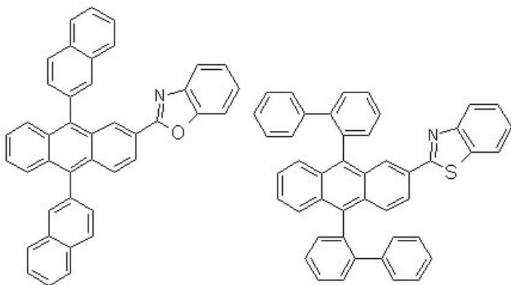
[화학식 3-9]
