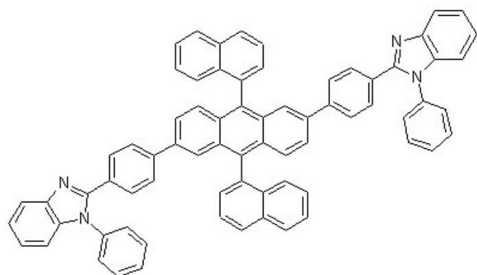
[화학식 2-4]
