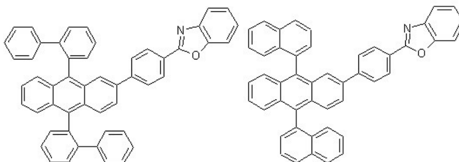
[화학식 1-11] [화학식 1-12]
