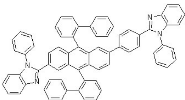
[화학식 5-3]
