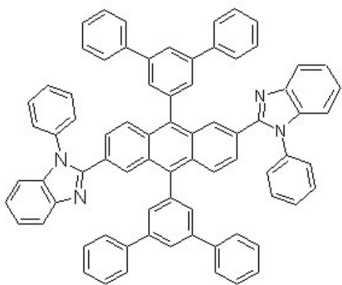
[화학식 4-5]
