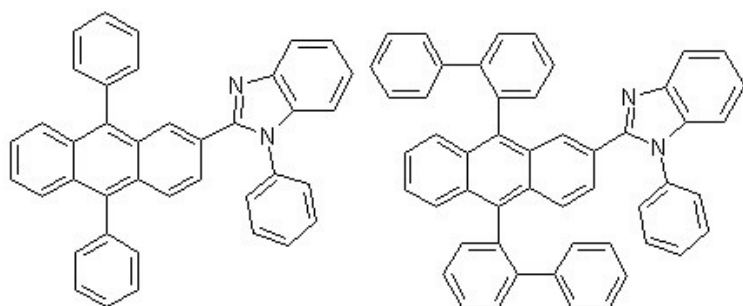
[화학식 3-3] [화학식 3-4]
