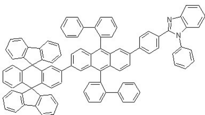
[화학식 1-15]
