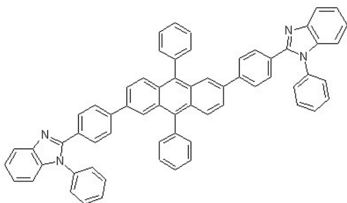
[화학식 2-2]
