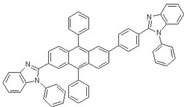
[화학식 5-2]
