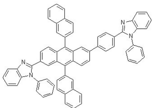
[화학식 5-5]
