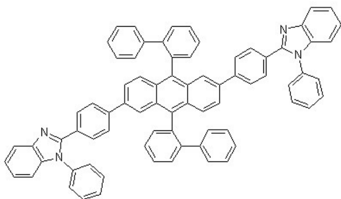
[화학식 2-3]
