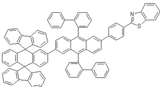
[화학식 1-16]
