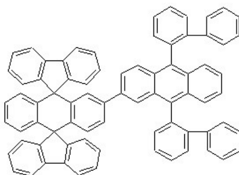
[화학식 l]
