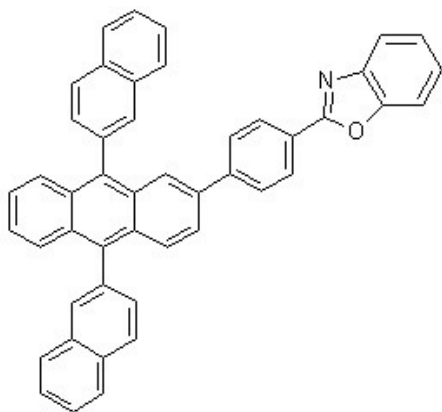
[화학식 1-14]
