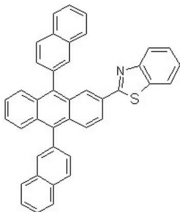
[화학식 3-9]
