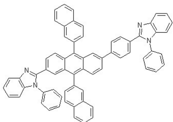
[화학식 5-5]
