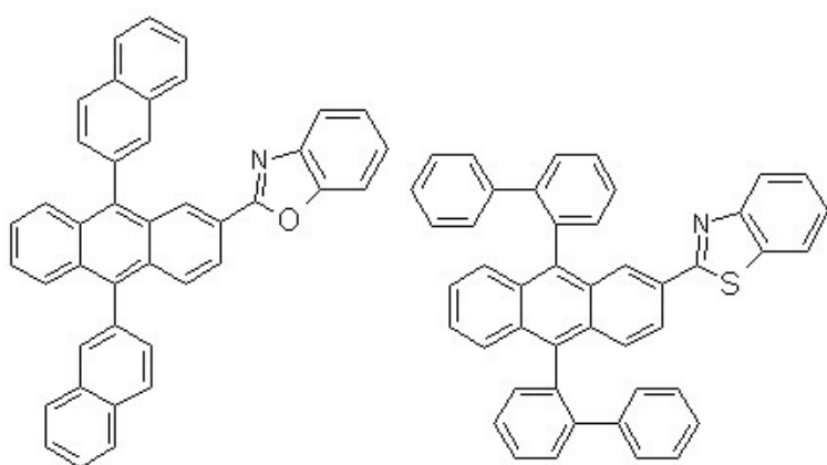
[화학식 3-9]
