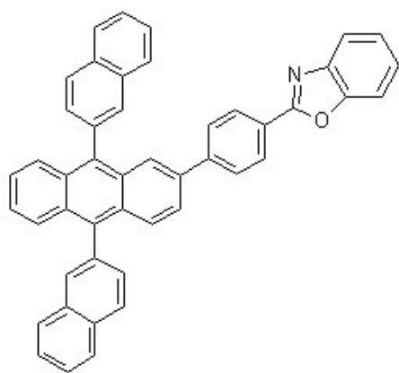
[화학식 1-14]
