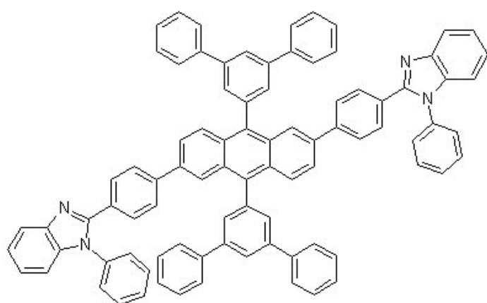
[화학식 3-1] [화학식 3-2]
