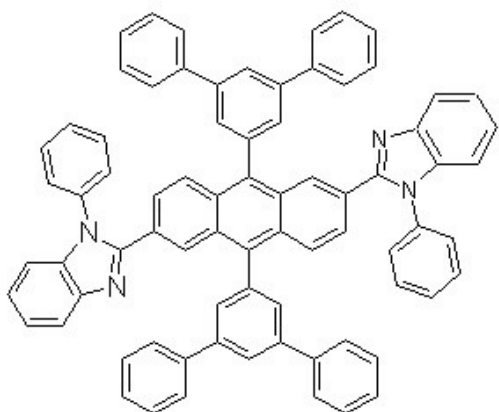
[화학식 4-5]
