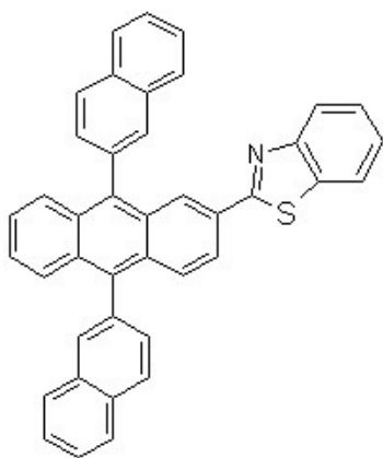
[화학식 4-1] [화학식 4-2]
