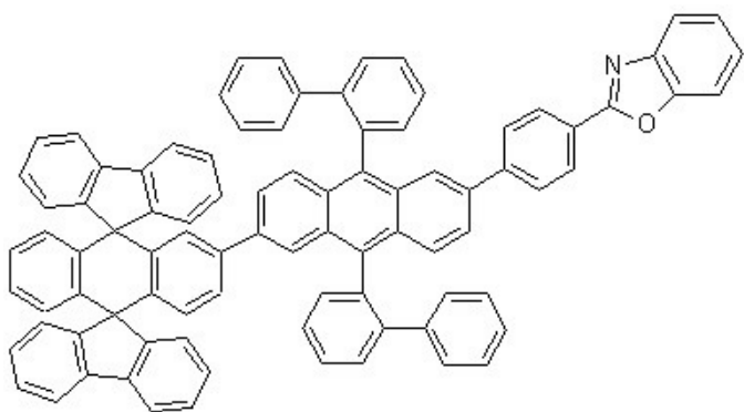
[화학식 1-16]
