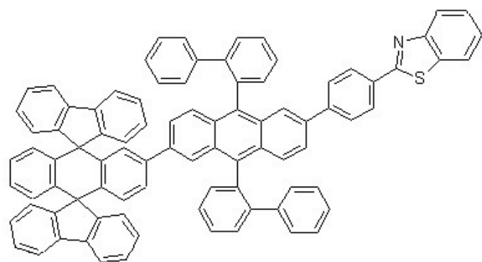
[화학식 1-16]
