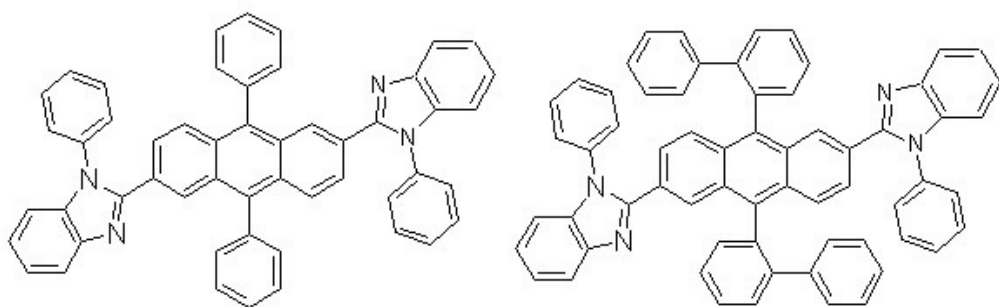
[화학식 4-3] [화학식 4-4]
