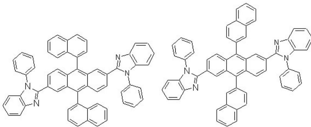
[화학식 4-3] [화학식 4-4]
