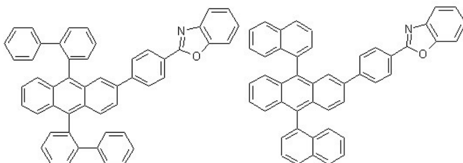
[화학식 1-11] [화학식 1-12]
