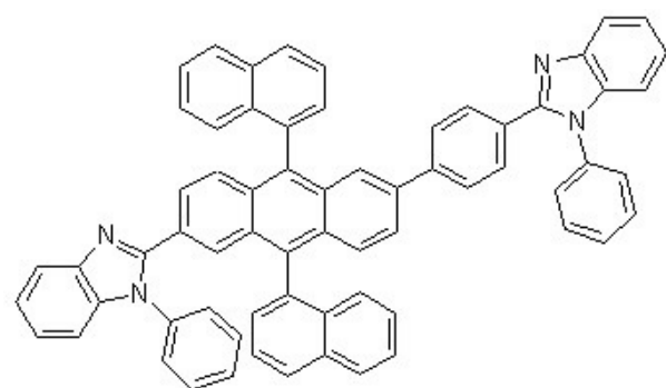
[화학식 5-4]
