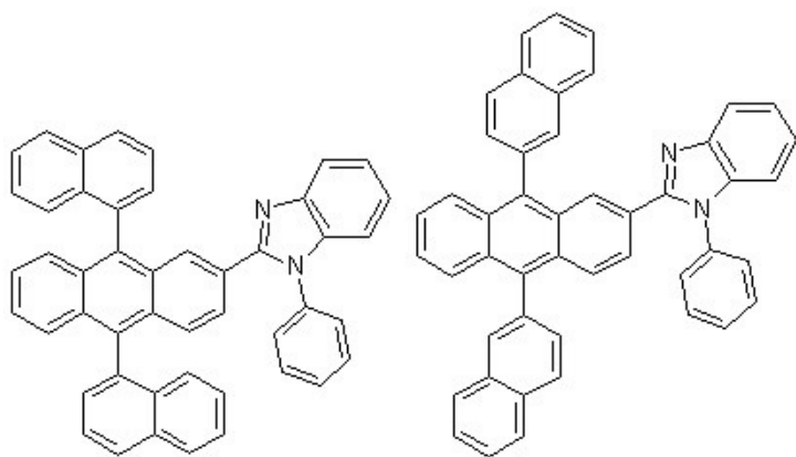
[화학식 3-5] [화학식 3-6]
