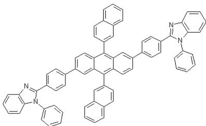
[화학식 2-5]
