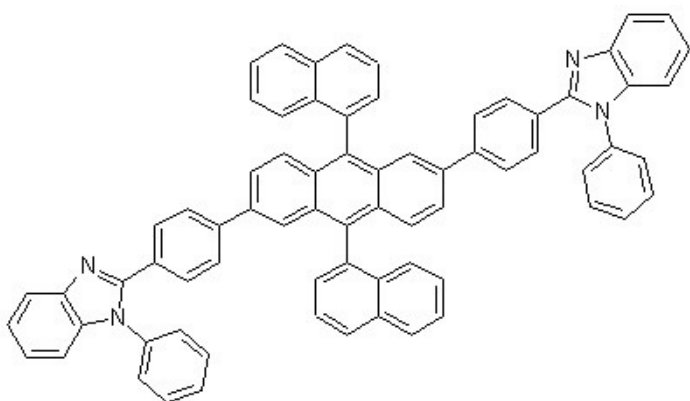
[화학식 2-4]
