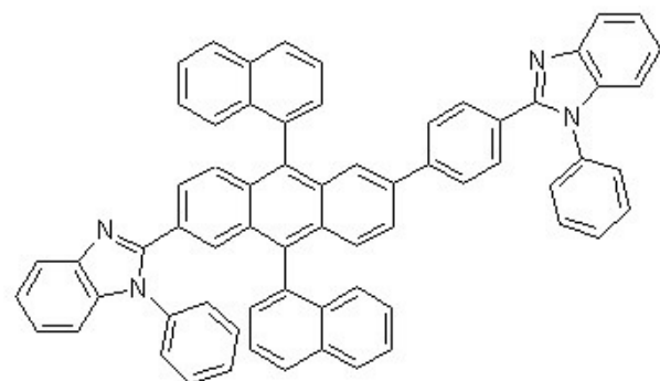
[화학식 5-4]
