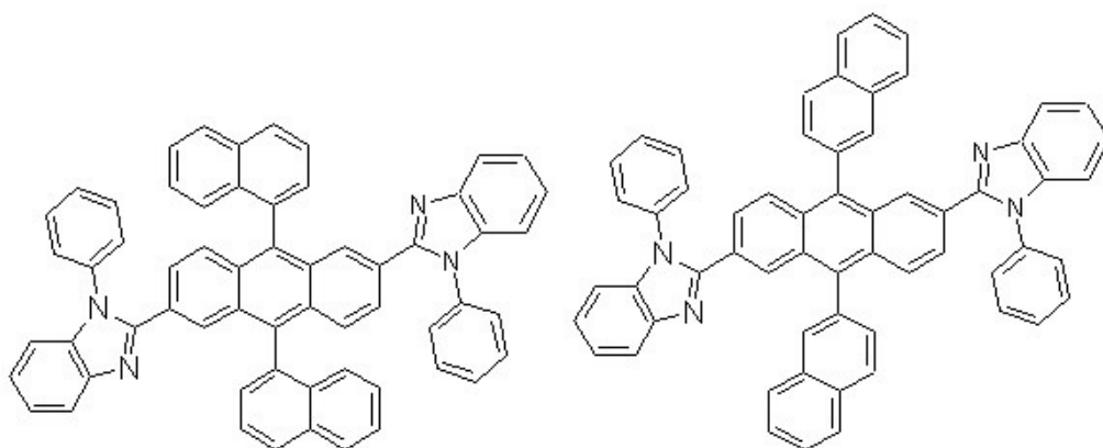
[화학식 4-3] [화학식 4-4]
