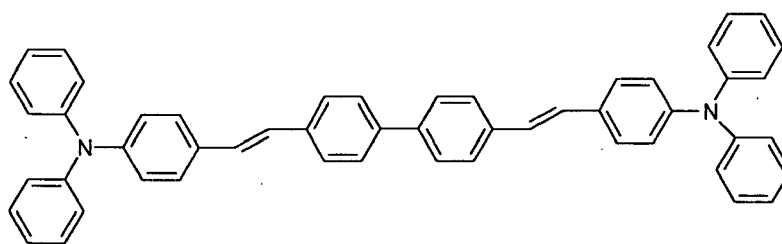
DSA amine
